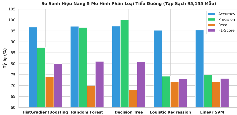
Figure 2.4: Biểu đồ so sánh đa chỉ số giữa 5 thuật toán phân loại tiêu đường
